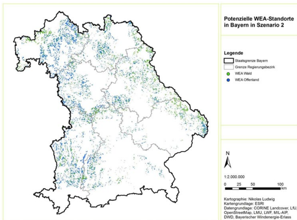
Abb. 10 Potenzielle Standorte von Windenergieanlagen (Szenario 2)
